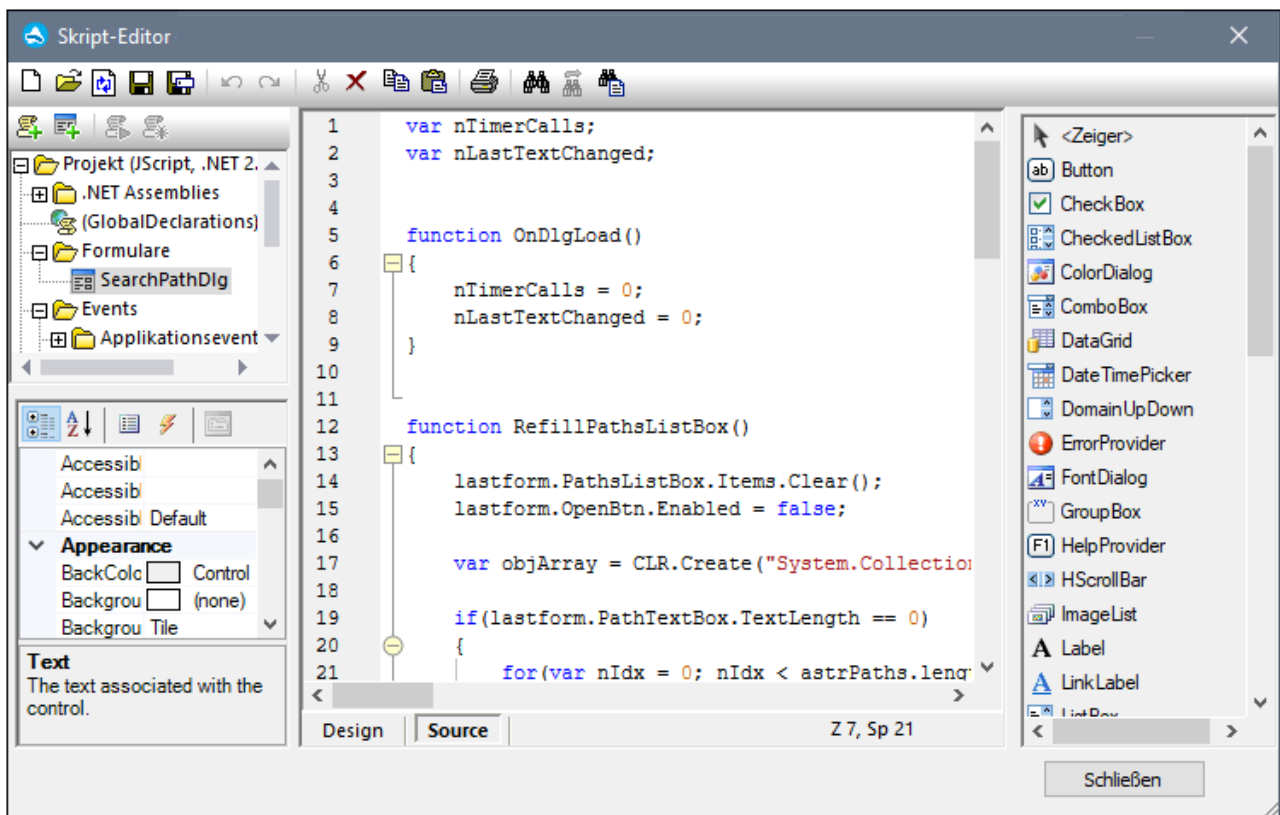
Skript-Editor
